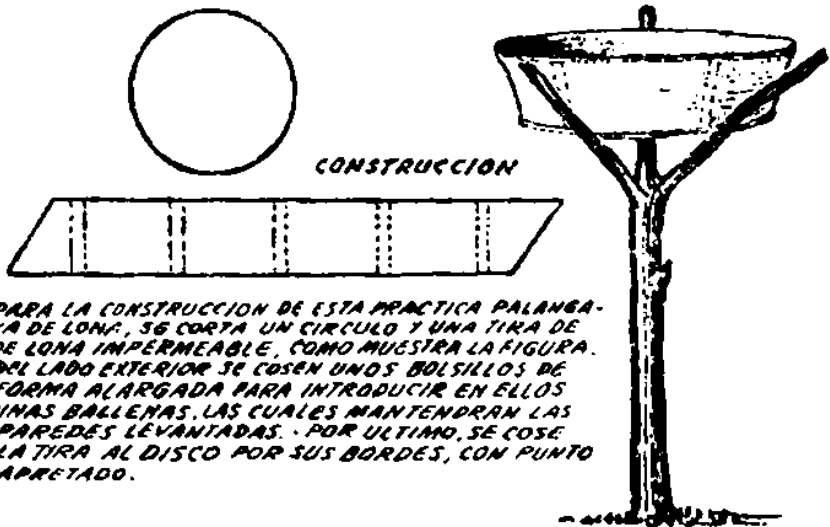
PALANGANA CONSTRUIDA EN CASA
