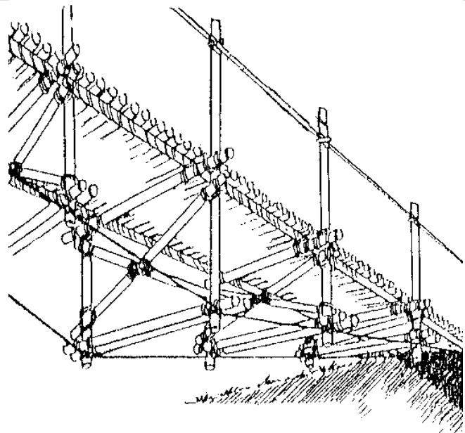
ESTA CLASE DE PUENTE SE CONSTRUYE SOBRE ESPACIOS MUY ENCAJONADOS Y TODO SU SISTEMA DE APOYO SE ENCUENTRA POR DEBAJO DEL PISO
