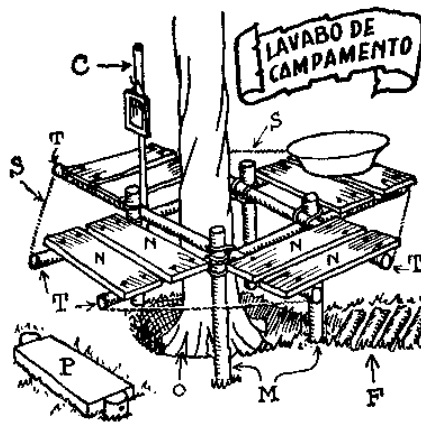
LAVADERO PARA 4 ACAMPANTES
