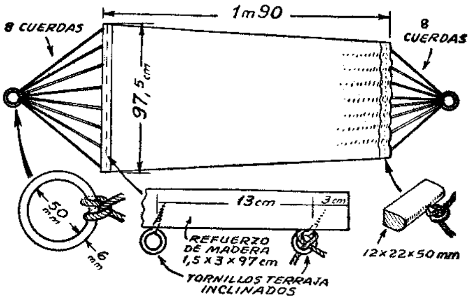
HAMACA PARA HACER EN CASA Y LLEVARLA A TODOS LADOS
